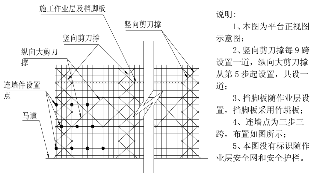
图 3.2-3 施工平台正视图
