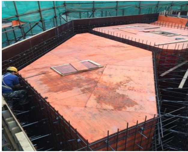
图 5.4-5 空箱模板安装预留人孔洞图
