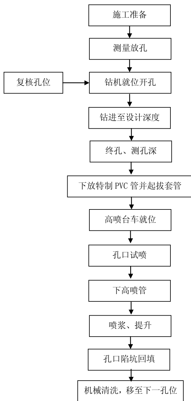
图 2.2-2 高压旋喷施工流程图
