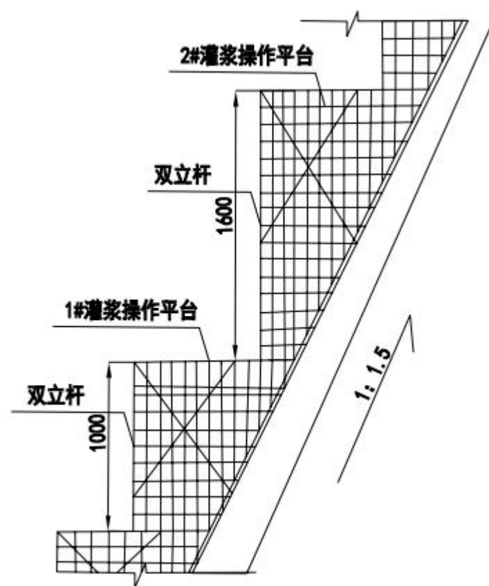
图 3.2-3 施工平台正视图
