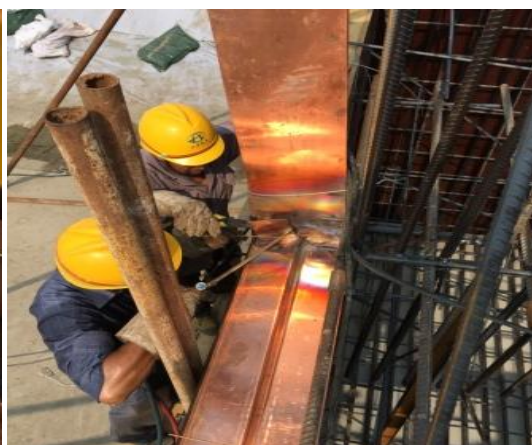
图 5.1-11 垂直铜止水焊接
