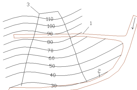
图 3.1-7 岸坡集中式道路布置示意图
