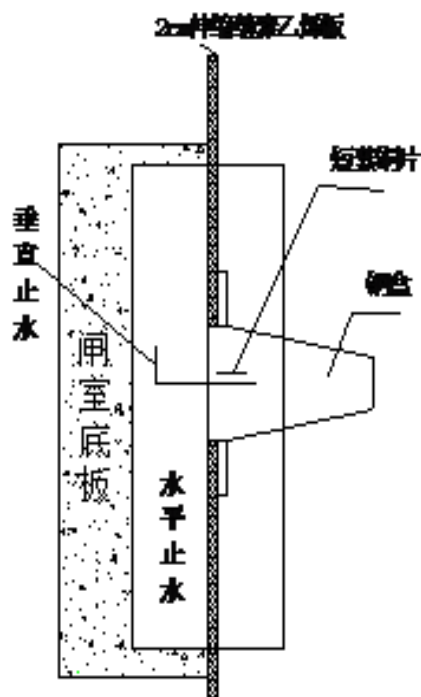
图 5.1-13 底板与墙身衔接处止水布置图
