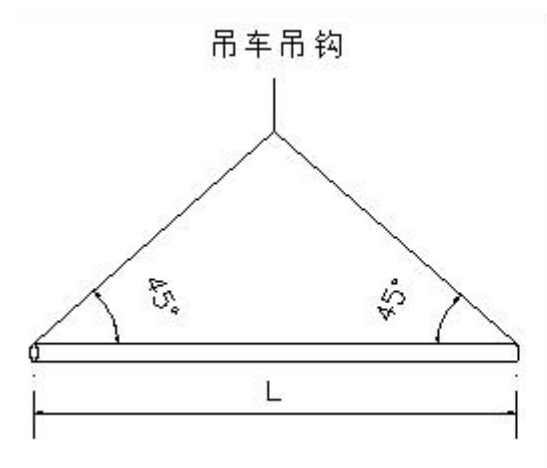
图 4.2-5 两头勾吊法吊运管桩示意图
