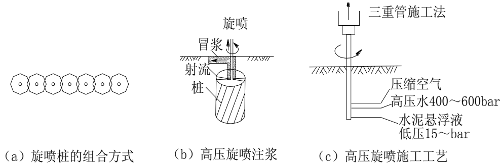
图 2.2-1 高压旋喷工艺示意图
