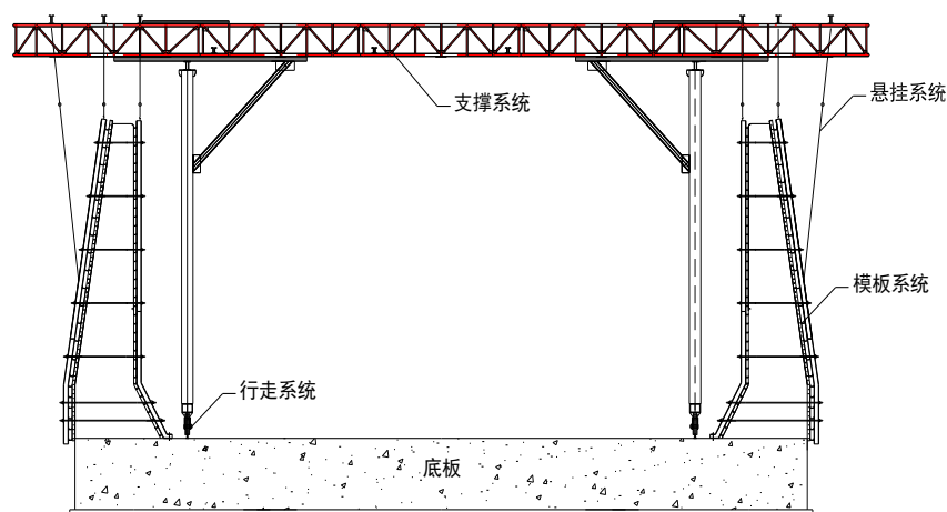
图 5.2-7 闸室墙模板龙门支架
