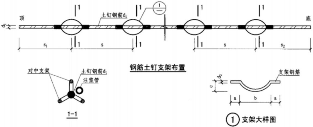
图 3.2-5 锚杆中心定位支架示意图
