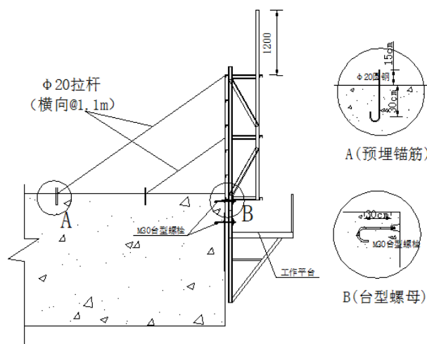
图 5.2-12 模板与工作平台安装与加固图
