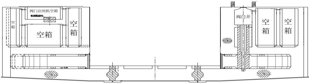
图 5.4-1 闸首边墩结构形式
