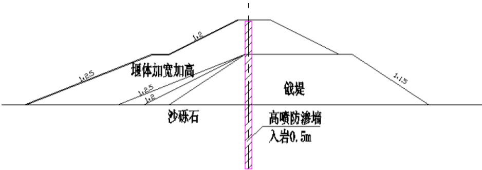
图 2.1-1 土石围堰结构断面
