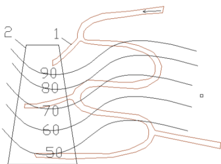
图 3.1-8 岸坡迂回式道路布置示意图
